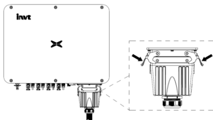
图 5.7 AC 防水罩卡扣固定
