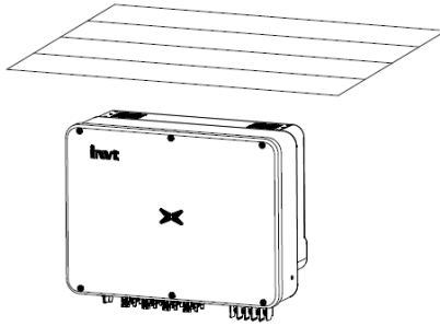
图 4.2 遮阳棚
