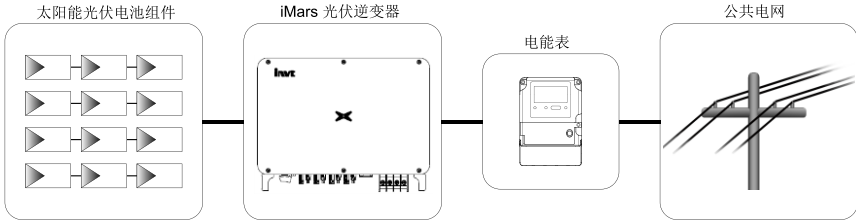
图 2.1 光伏并网逆变器应用
