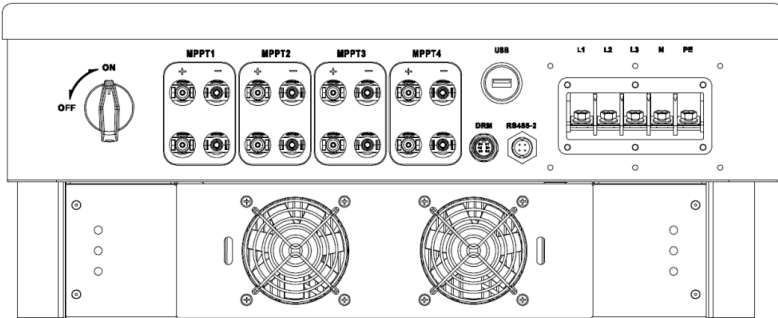
XG25-40KTR 底部示意图
