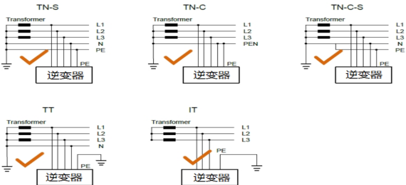
图 2.2 光伏并网逆变器支持的电网形式
