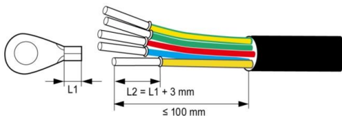
图 5.5 压接电缆端子
