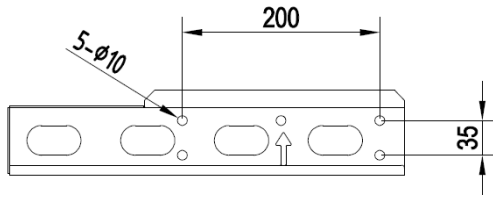
图 4.6 安装挂板尺寸图
